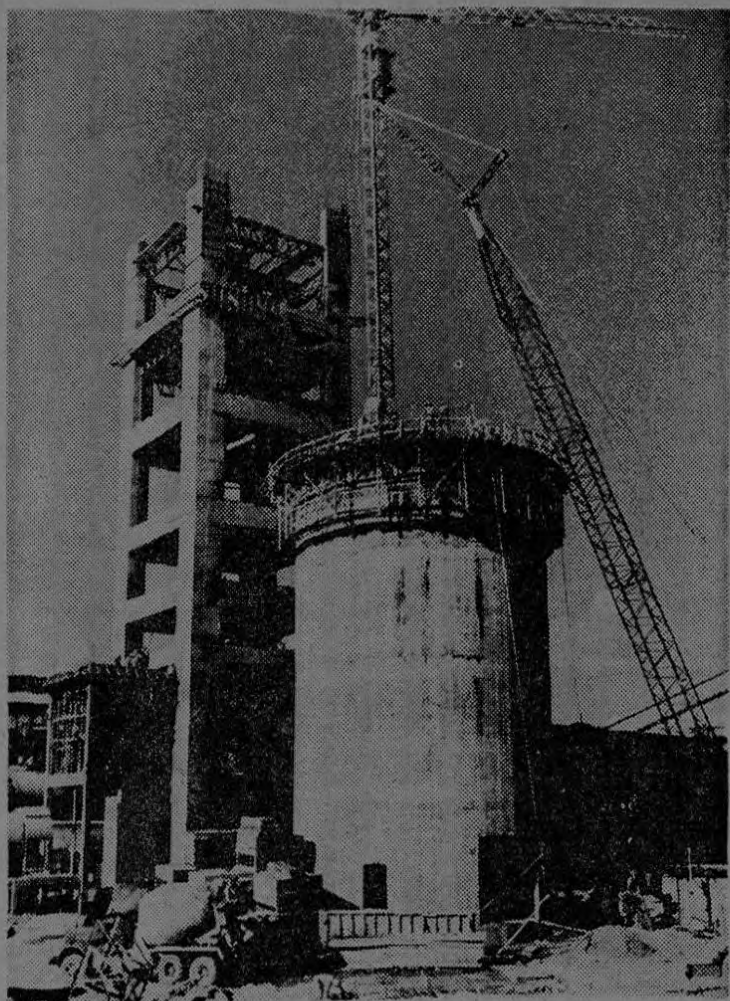
Aspecto de la construcción de la Torre de pre-calentamiento y silo de materia prima, al 30 de Abril, 1970.
